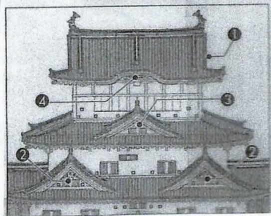
①入母屋破風 ②比翼入母屋破風 ③千鳥破風 ④軒唐破風 ⑤切妻破風
